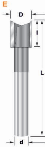
5105 HSS C05 κοντύλια αλουμινίου / single flute cutters A Z1
