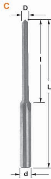
9-9D HM κοντύλια ελικοειδή για αλουμίνιο και πλαστικό / solid carbide spiral router for AL and plastic F
