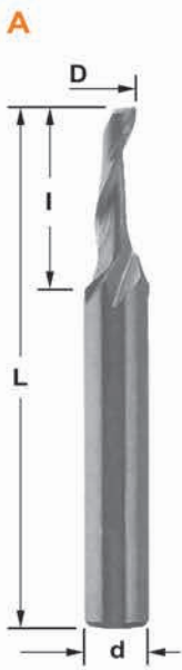
5105 HSS C05 κοντύλια αλουμινίου / single flute cutters A Z1
