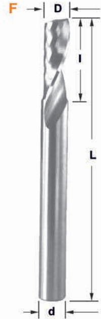
9-9D HM κοντύλια ελικοειδή για αλουμίνιο και πλαστικό / solid carbide spiral router for AL and plastic F
