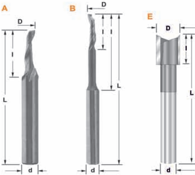
5105 HSS C05 κοντύλια αλουμινίου / single flute cutters
