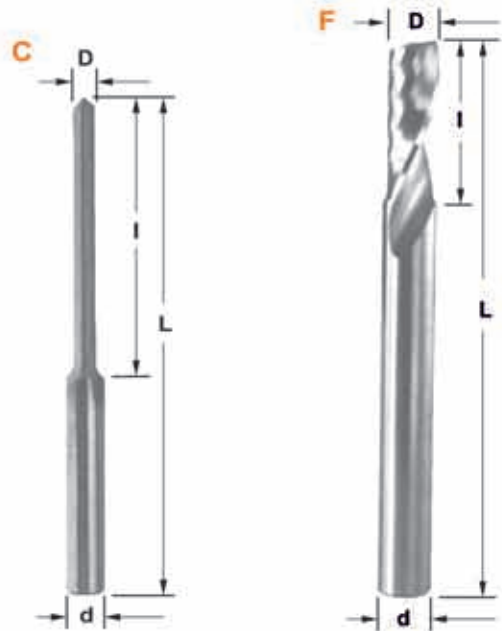
9-9D HM κοντύλια ελικοειδή για αλουμίνιο και πλαστικό / solid carbide spiral router for AL and plastic
