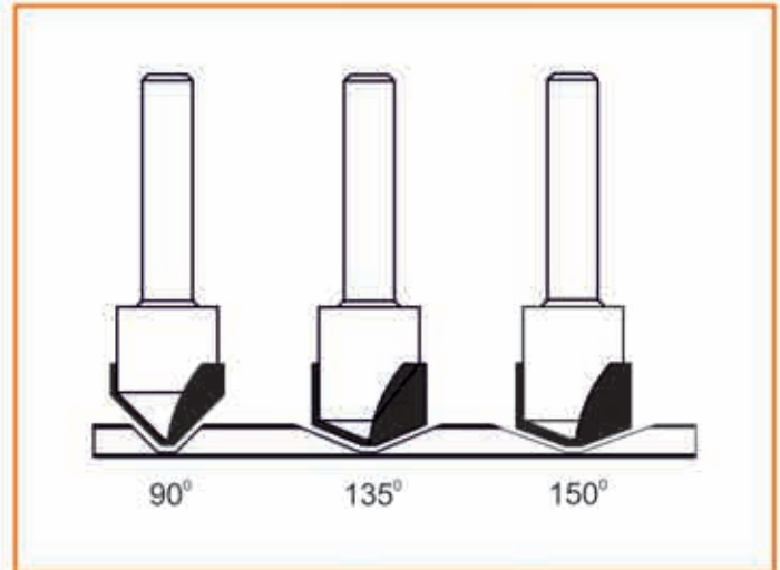
5105 Κοντύλια ETALBOND-ALUCOBOND ETALBOND-ALUCOBOND routers
